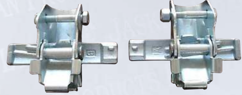
MODEL: JPPL-1619 A,B WEDGE CLAMP LEFT RIHGT
