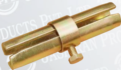
MODEL: JPPL-607 JOINT PIN (EN 74/ BS 1139)
